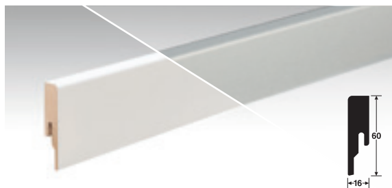
Akzent-Sockelleiste ASL 60 (weiß, dekoridentisch, edelstahl, anthrazit, schwarz) 16 x 60 x 2380 mm
